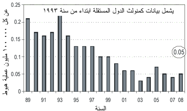
عدد الحوادث المميتة عن كل ١٠٠,٠٠٠ مليون عملية هبوط لطائرات على الخطوط المنتظمة
