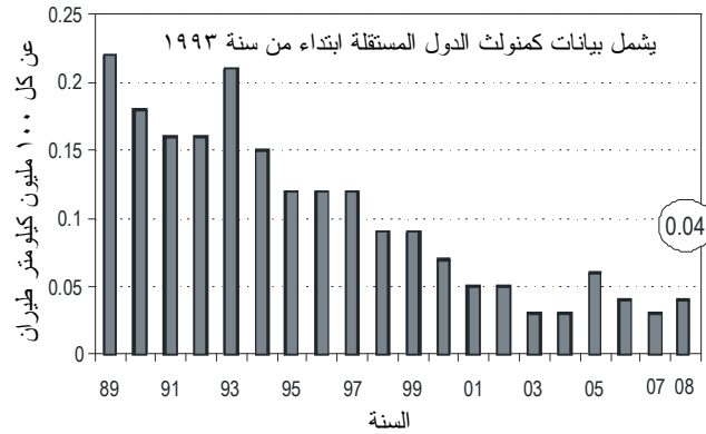
عدد الحوادث المميتة عن كل ١٠٠ مليون كيلومتر طيران على الخطوط المنتظمة
