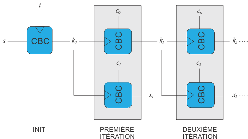
Figure 2. Mappage de nombres pseudo-aléatoires
