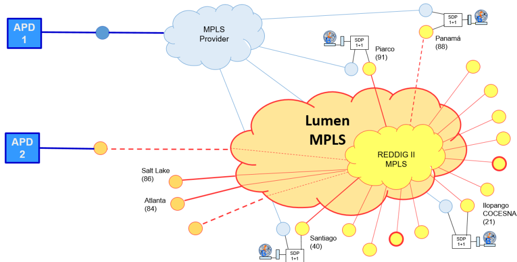
Figura 1 – Red IP regional (REDDIG II) como enlace de distribución de ADS-B Satelital
