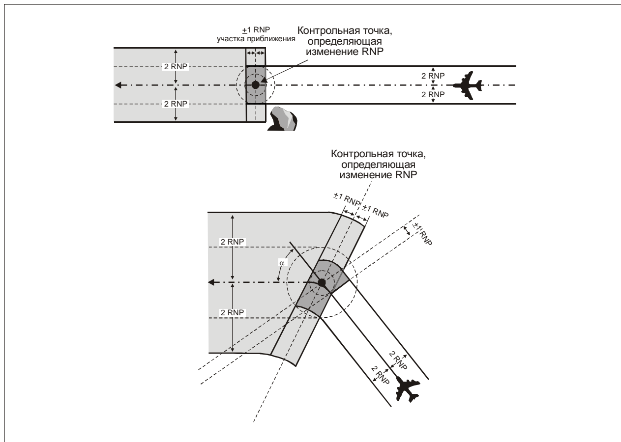
Рис. 4-4. Увеличение значения RNP (прямолинейный и криволинейный участки)
