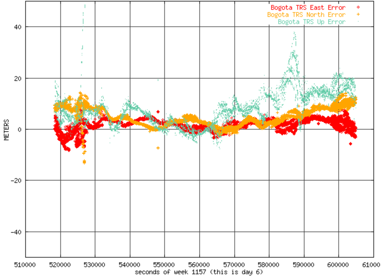
Figura 32. Error horizontal y vertical tomado de muestras de señal GPS - Colombia
