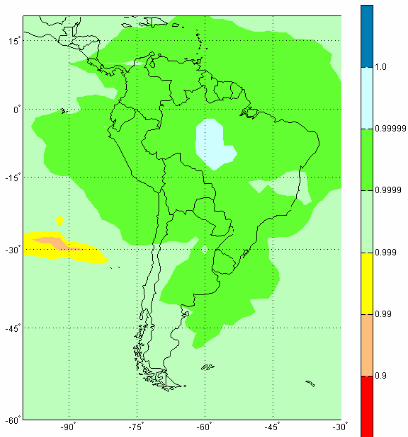
Figura 6a: Disponibilidad LNAV que ofrece el SAAS por sí solo con centelleo promedio (GPS 24 con fallas estocásticas) centelleo en la percentila 50. SAAS con 13 WRS.
