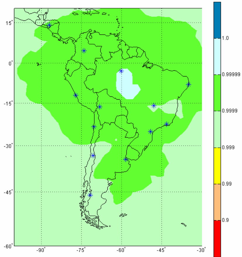
Figura 3a: Disponibilidad LNAV que ofrece el SAAS por sí solo (13 WRS) (GPS 24 con fallas estocásticas). No se ha modelado el efecto del centelleo. 13 WRS aparecen mostrados en color azul *.
