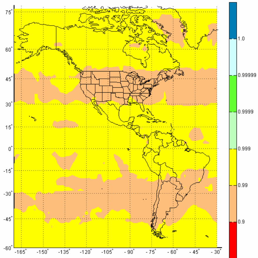
Figura 1a: Disponibilidad LNAV de la RAIM (GPS 24 con fallas estocásticas en el receptor SBAS). No se ha modelado el efecto de centelleo.
