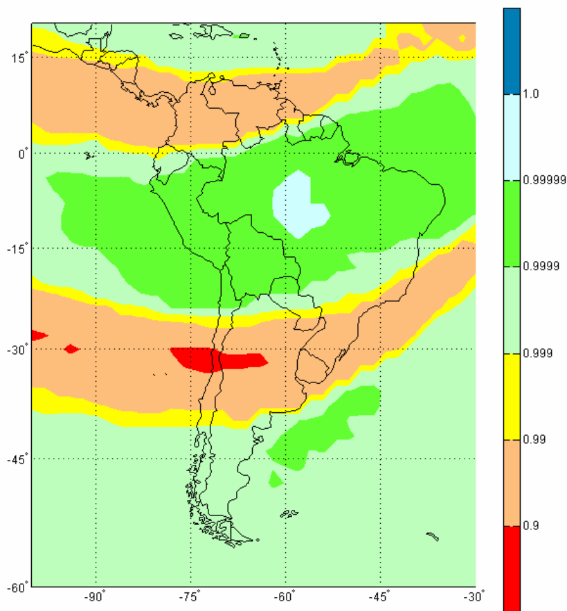
Figura 6b: Disponibilidad LNAV que ofrece el SAAS por sí solo con centelleo promedio (GPS 24 con fallas estocásticas) centelleo en la percentila 95. SAAS con 13 WRS.
