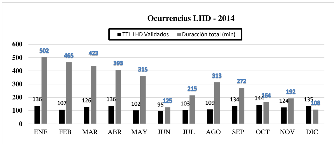
Gráfico 1. Ocurrencias/Duración de los LHD por Mes
