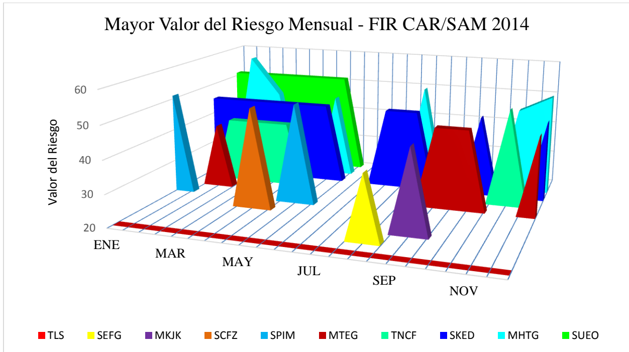
Gráfico 5. Mayor valor de riesgo para las FIR del espacio RVSM CARSAM. La línea roja es el VR de la TLS (20).
