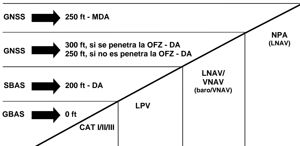
Figura 1 – Mínimos de aproximaciones GNSS
