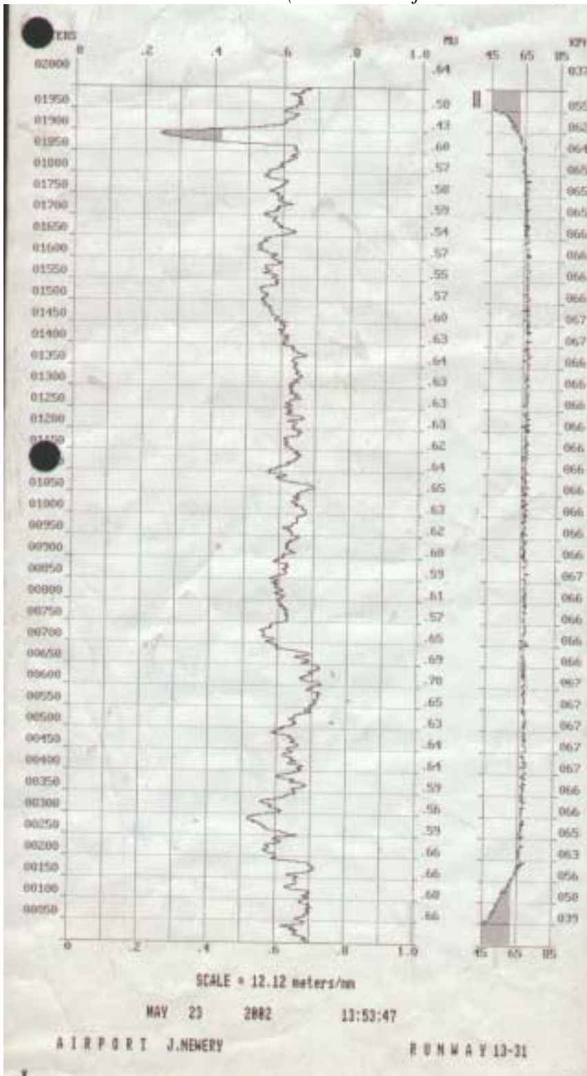
RGM del mes de mayo de 2002 (a seis meses de ejecutado el ranurado, sin haberse realizado descontaminación de caucho)
