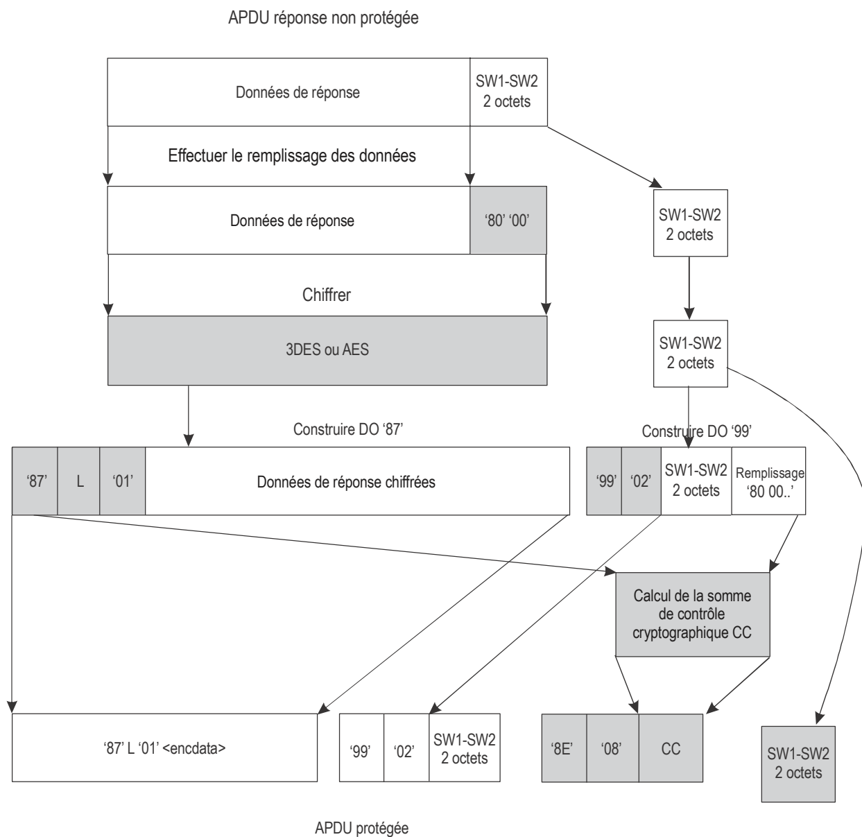
Figure 6. Calcul d'une APDU réponse de SM pour un octet INS pair
