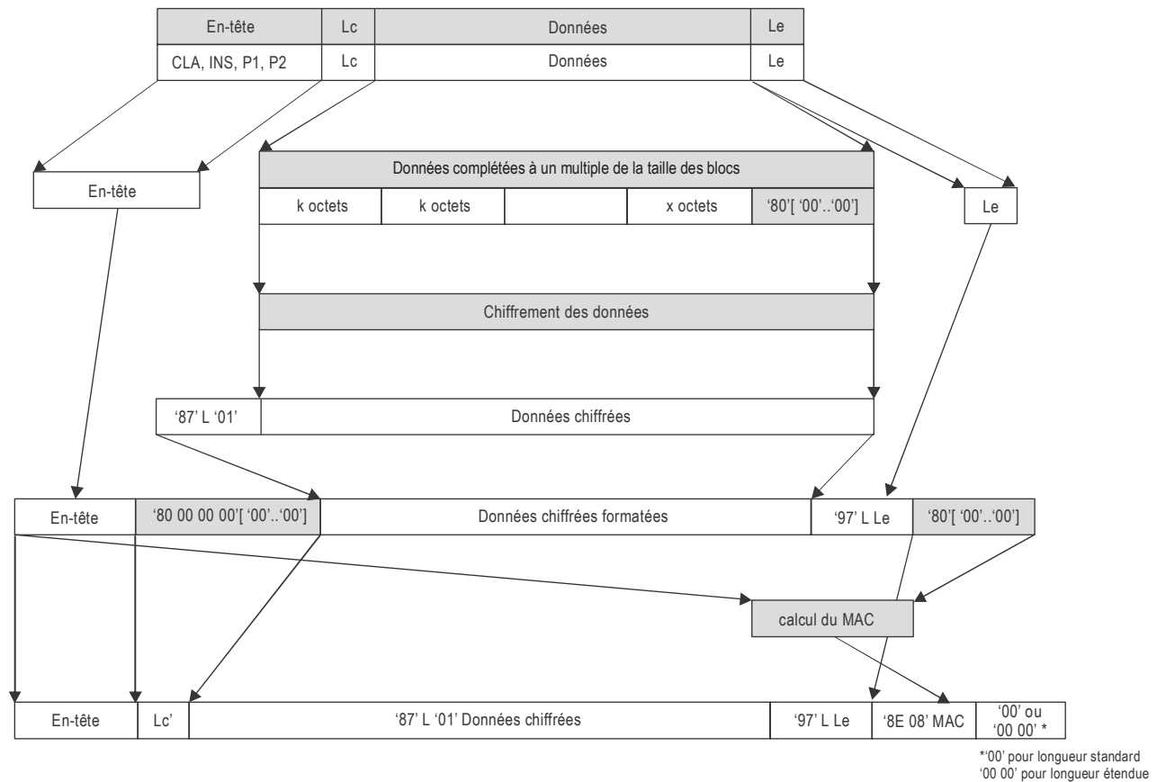
Figure 5. Calcul d'une APDU commande de SM pour un octet INS pair
