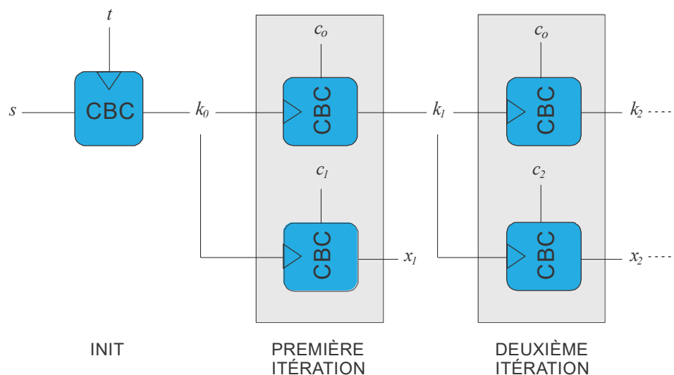
Figure 2. Mappage de nombres pseudo-aléatoires
