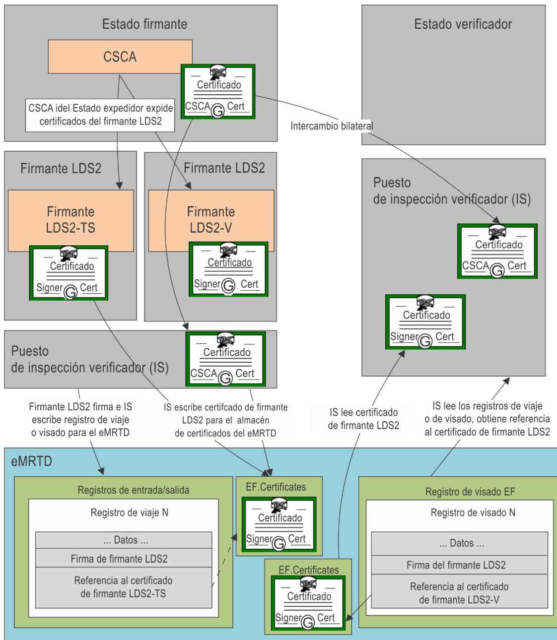
Figura G-1. Firma digital de la LDS
