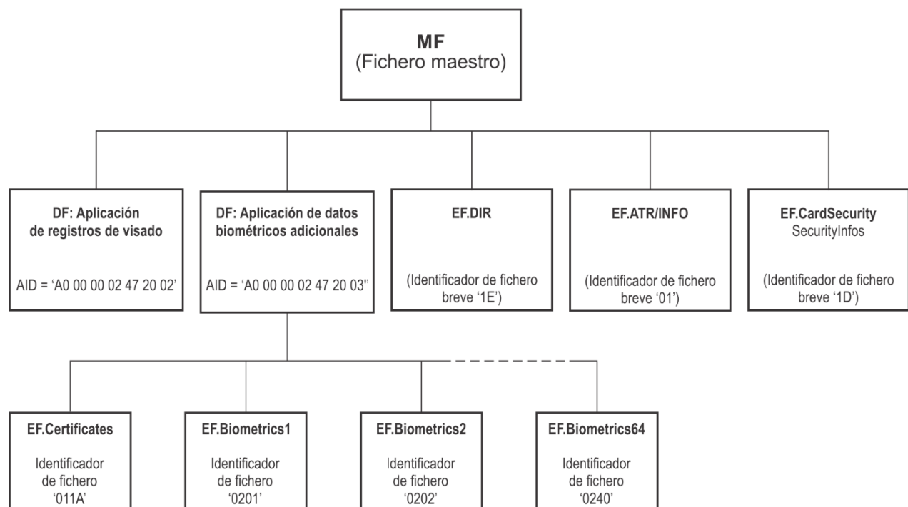
Figura 6. Estructura de la aplicación de los datos biométricos adicionales
