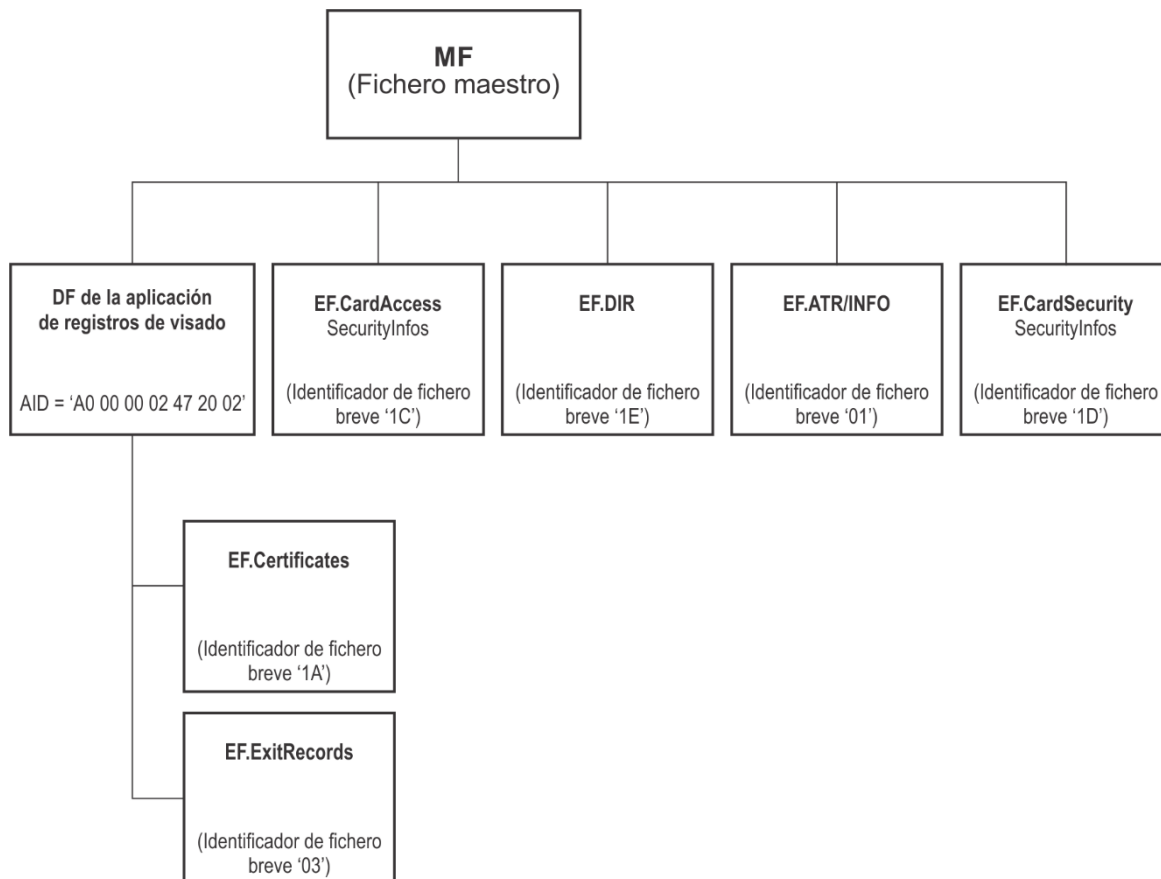
Figura 5. Estructura de los registros de visados
