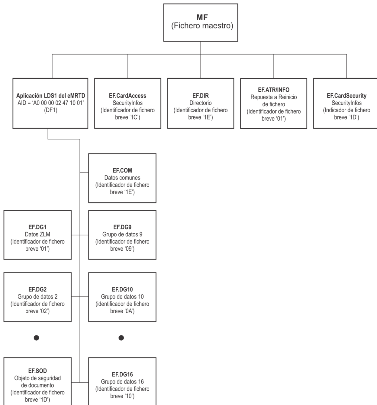
Figura 3. Resumen de la estructura de fichero de la LDS1 del eMRTD
