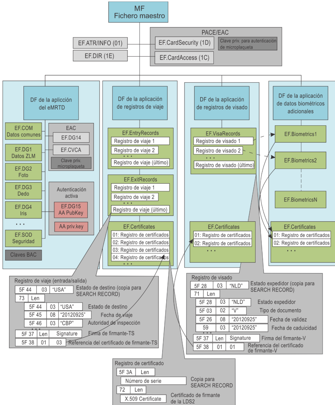
Figura E-1. Resumen de las estructuras de fichero
