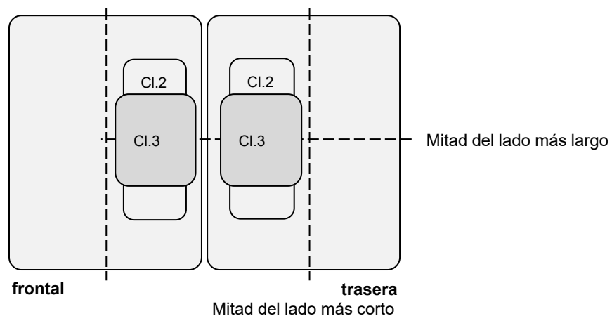
Figura C-1. Posiciones obligatorias en cada superficie de ID-3 en la que un sistema de inspección asociado a un eMRTD de tipo 1 y 2 leerá las antenas de clase 2 y 3
