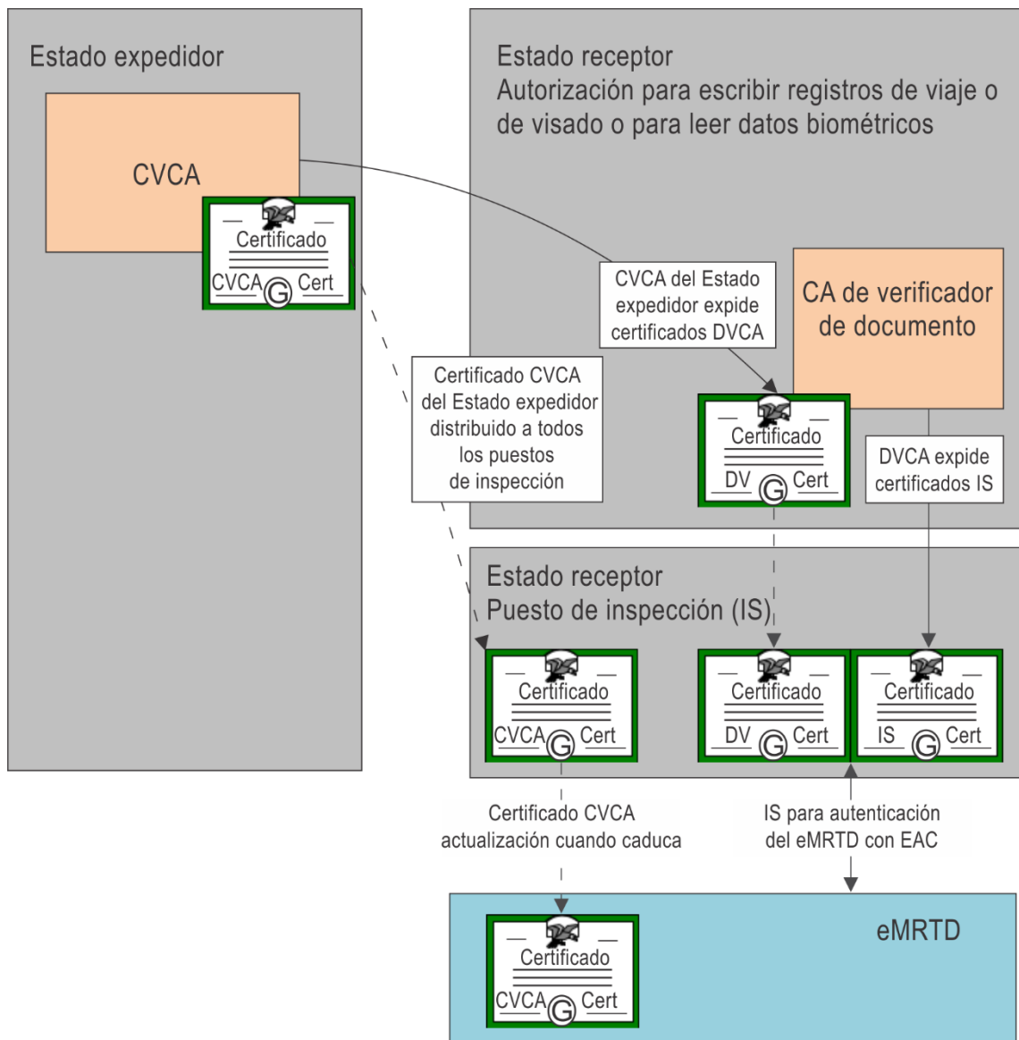
Figura F-1. Resumen de la autorización de la LDS
