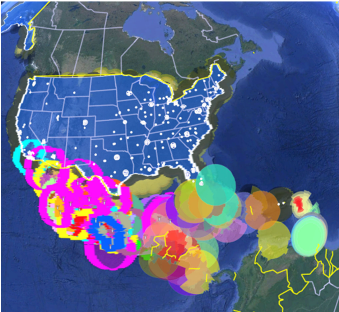
Figura 2. MAPA de cobertura ADS-B de los miembros NAM
