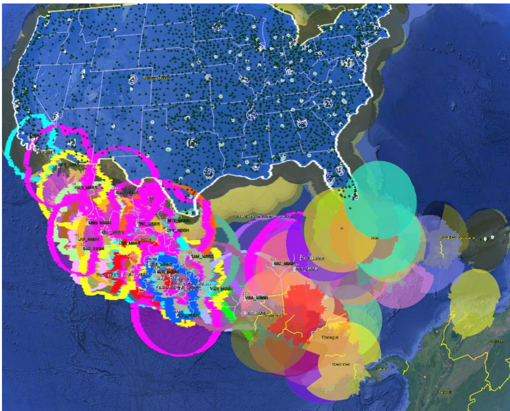
Figura 2. MAPA de cobertura ADS-B de los miembros NAM
