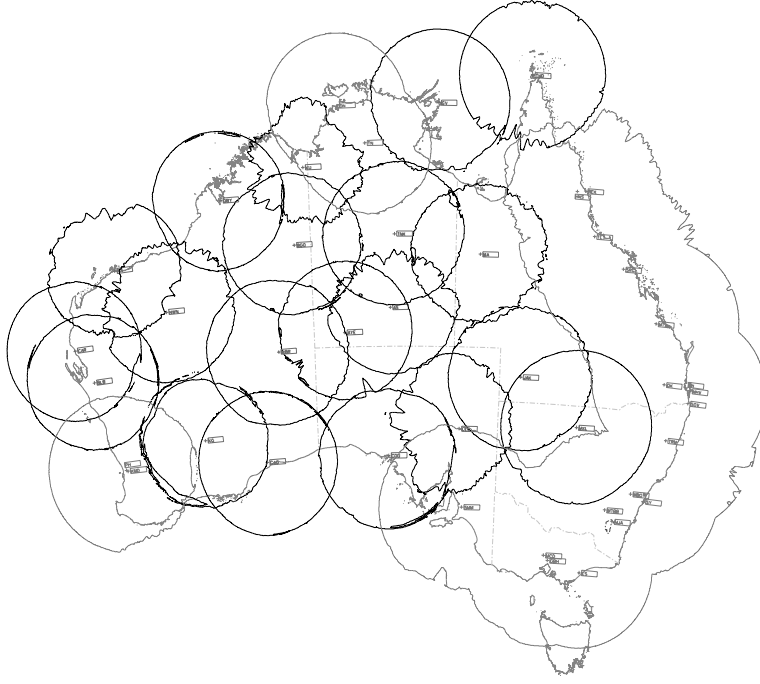
الشكل ٣ - الرادار المركب المقترح والتغطية بالاستطلاع التابع التلقائي-البث عند مستوى الطيران FL 300 بعد وزع ٢٠ موقفا للاستطلاع التابع التلقائي ADS-B.
