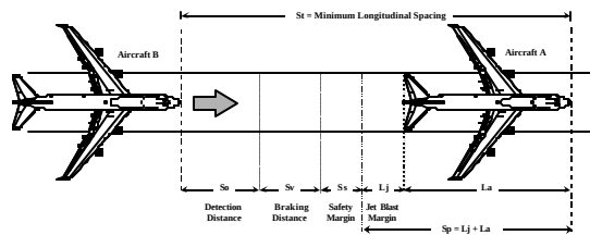
Figure 3-2. Longitudinal spacing parameters
