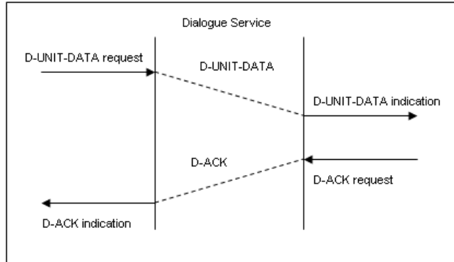
Figure 11. D-UNIT-DATA Service (UDP)
