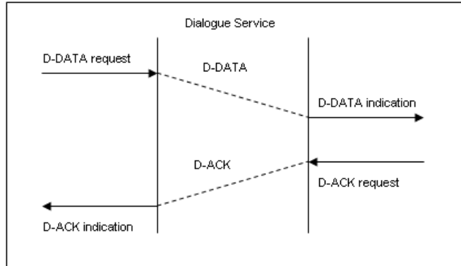
Figure 6. D-DATA Service (UDP)
