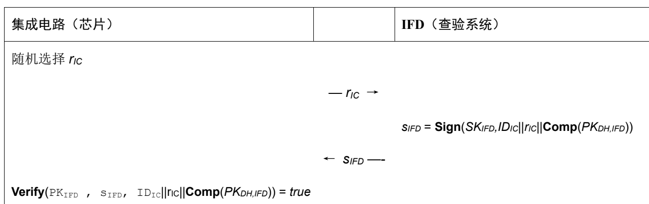
图 4. 终端认证
