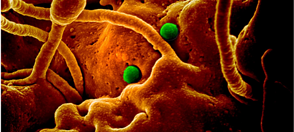
骆驼上皮细胞上的 PMERS-CoV 颗粒。国家过敏和传染病研究所 (NIAID) 与科罗拉多州立大学协作提供照片。
